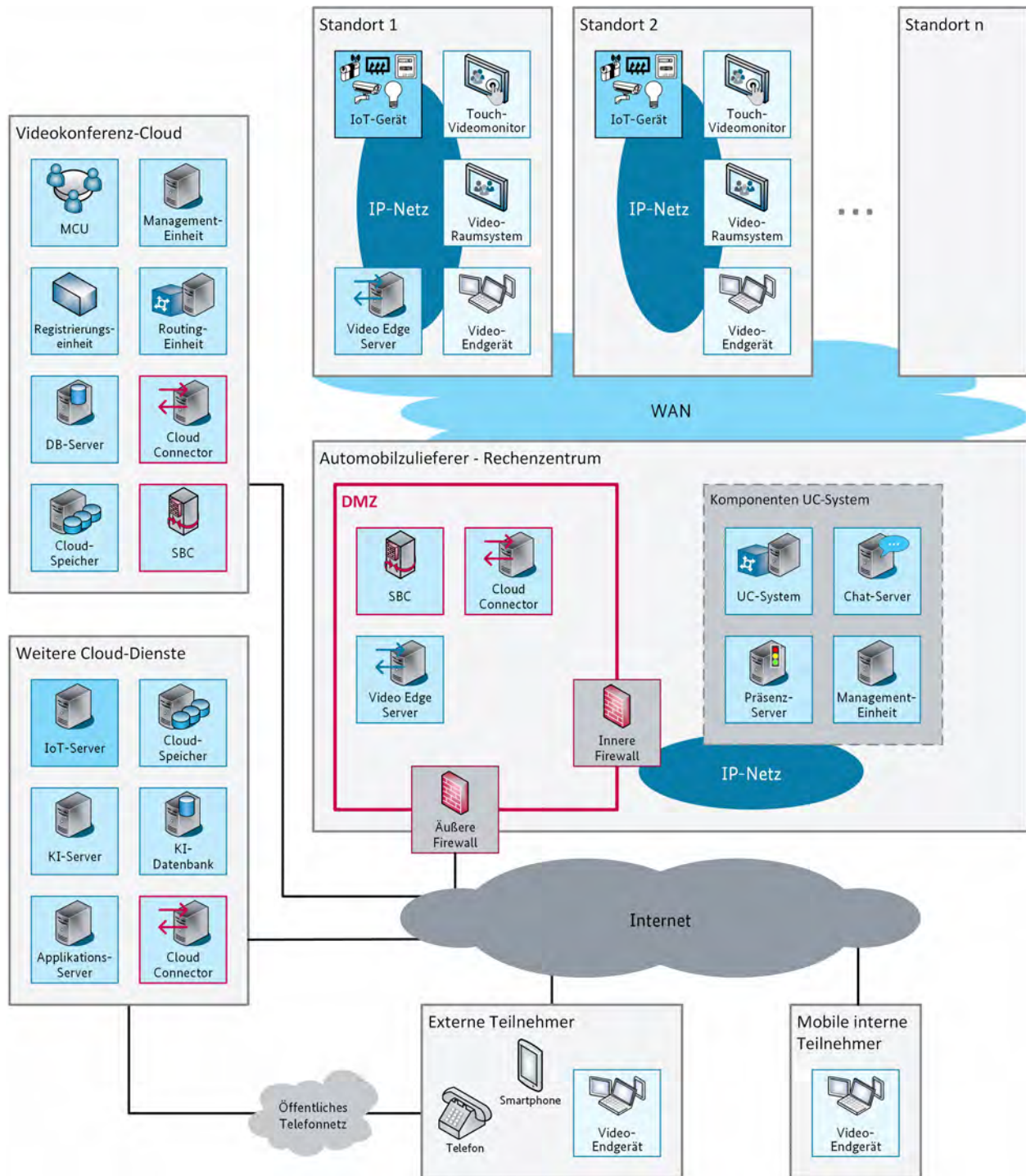
Abbildung 18: Hybrid-Lösung
